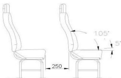
Figura 3 – Distâncias livres e ângulos de inclinação
